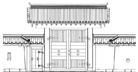
⑱西仕切門 (計画図)
